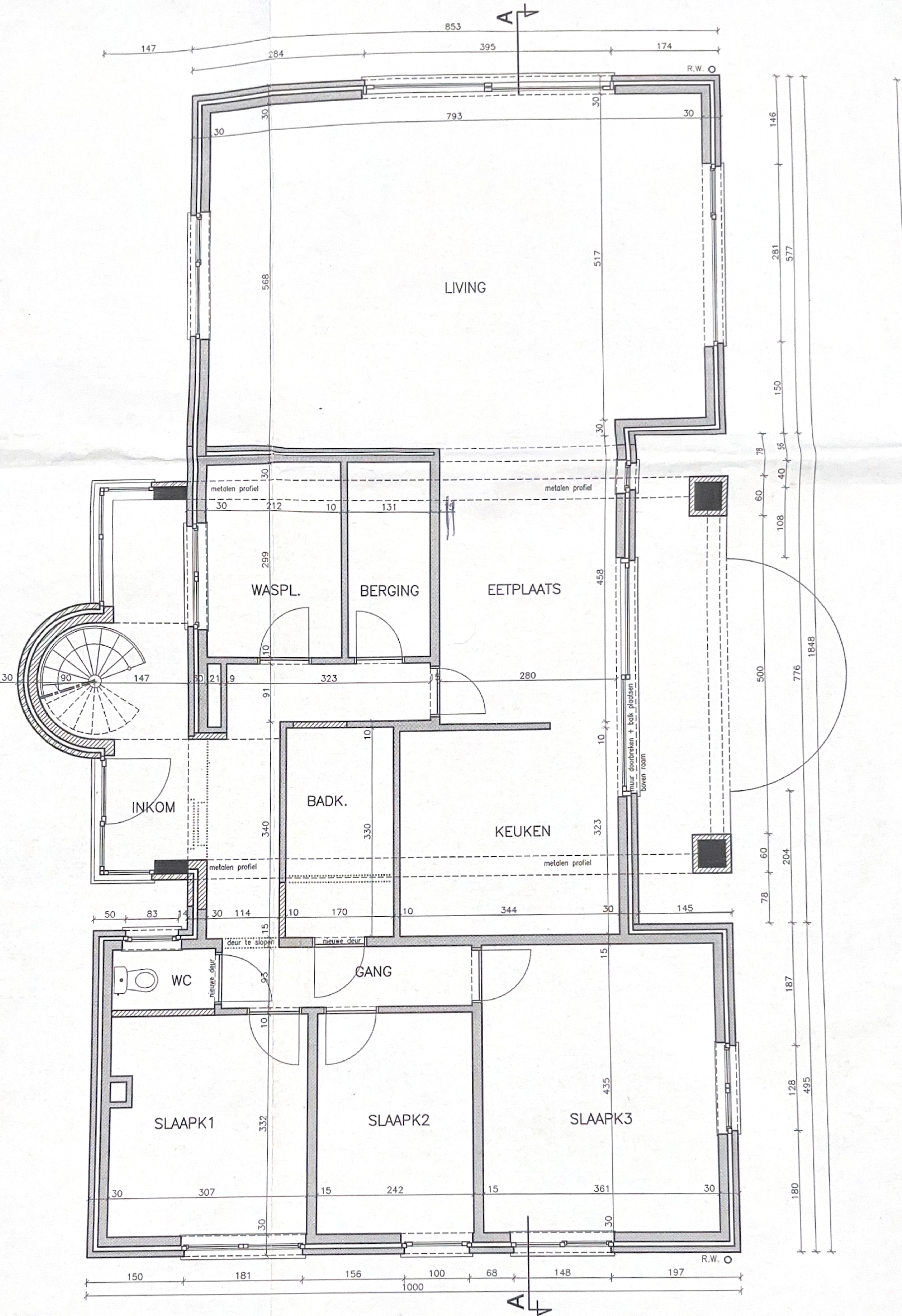
PLAN GELIJKVLOERS
